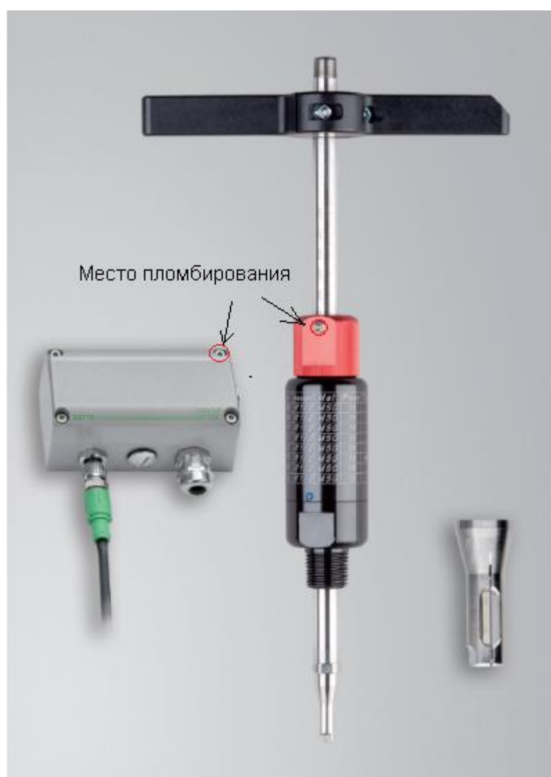
Рисунок 10 - Общий вид модели EE776
